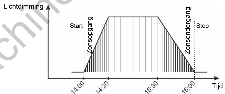
Figuur 10: Normaal licht dimmen Zonsopgang en zonsondergang zijn geïntegreerd in de lichtperiode.
