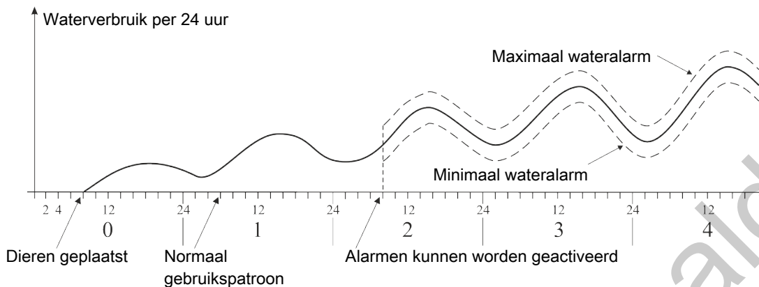
Figuur 14: Voorbeeld van minimaal en maximaal wateralarm
